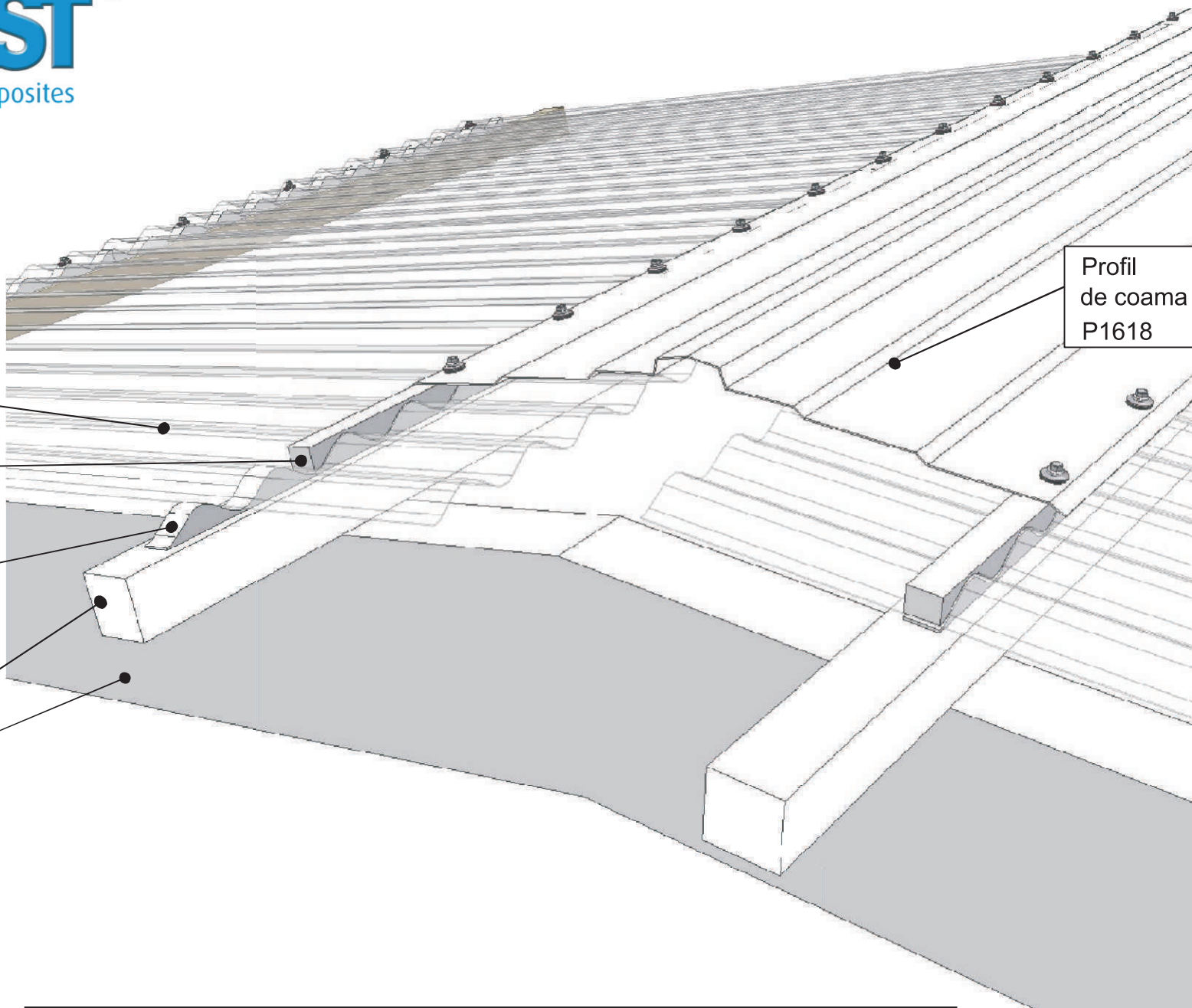
Instalare utilizand Profile de coama pentru Policarbonat P1618
